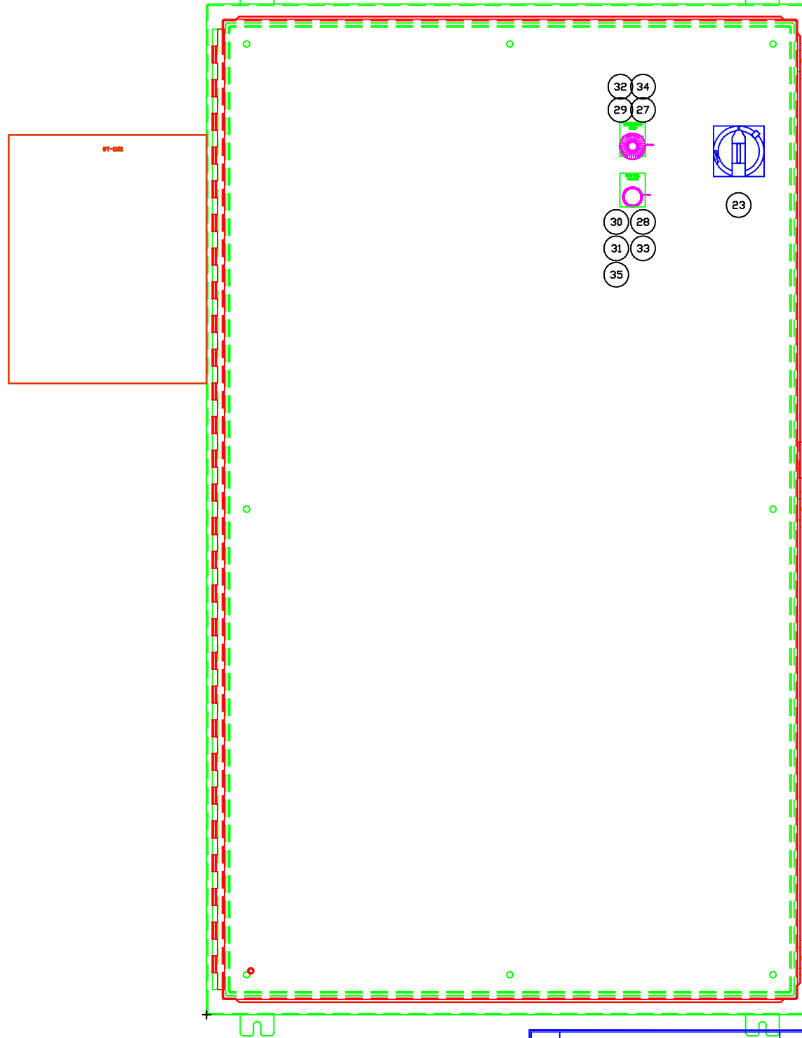
Door Scale: 1.5" = 1'-0"
